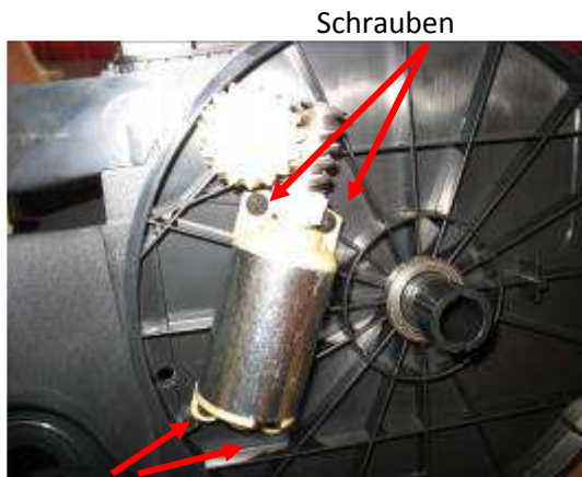
Schrauben
